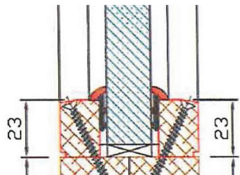
Exemple de mise en œuvre sur porte bois
